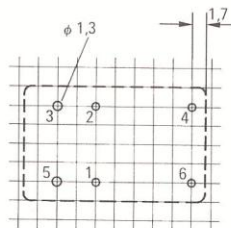
Montagelochung Ansicht auf die Anschlüsse
